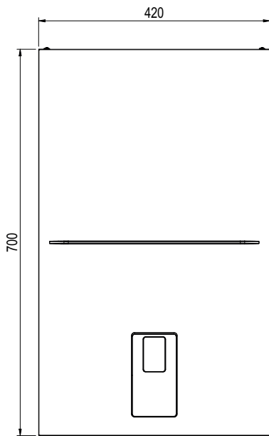
εικ. 70- Μπροστινή όψη
