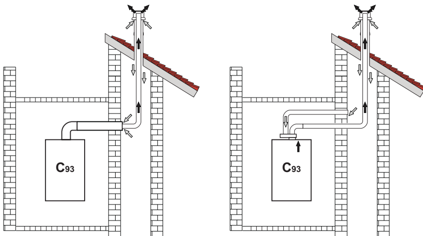
fig. 43- Ejemplos de conexión a chimeneas (⇨ = aire / ⇩ = humos)
