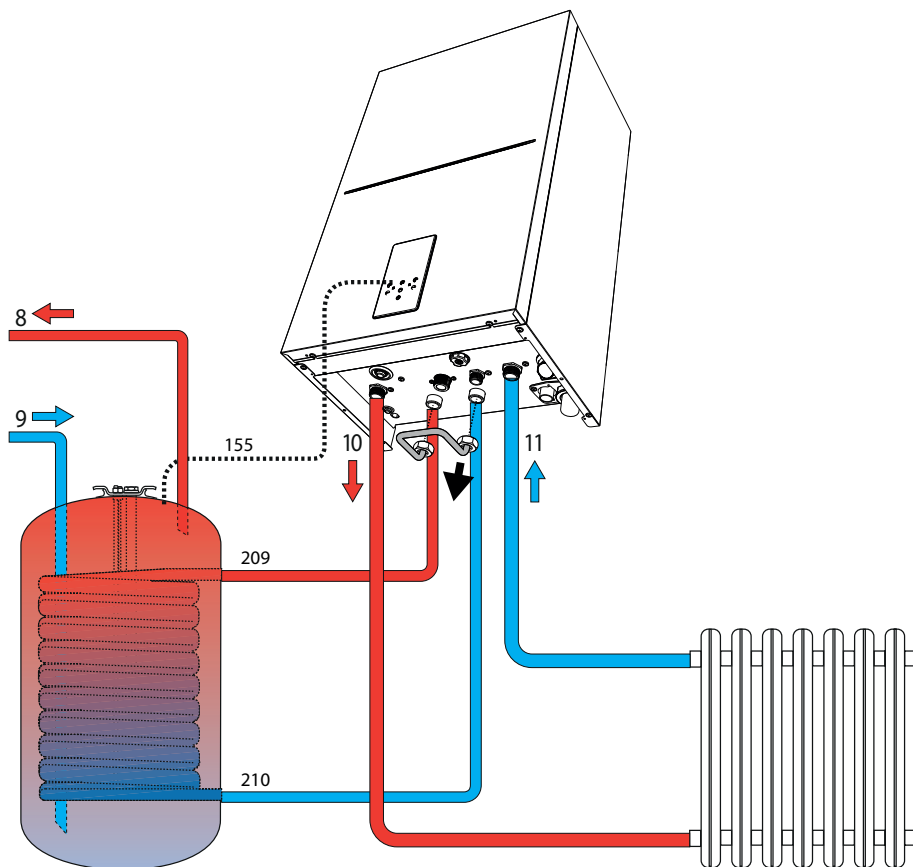
fig. 28- Esquema de conexión a un termotanque externo
