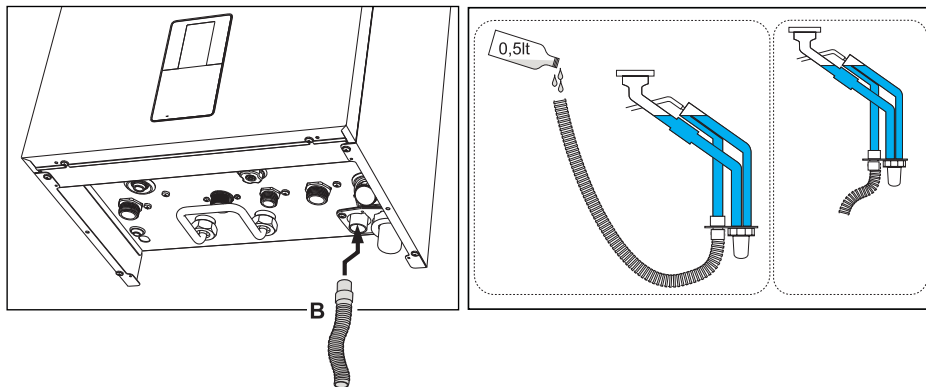
fig. 51- Racordarea evacuării condensului
