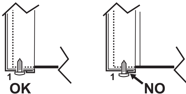
wygląd 56- Prawidłowe położenie przedniego panelu
