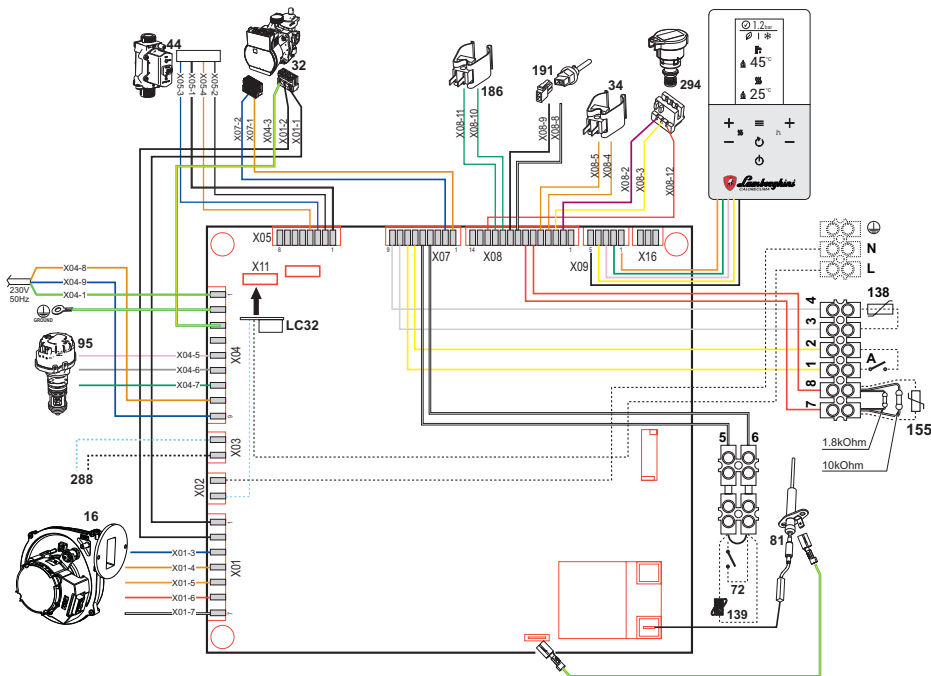
fig. 79- Schema electrică
