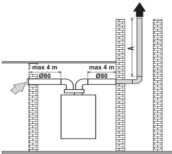
εικ. 39- Διάγραμμα μόνο για τοποθέτηση εύκαμπτου σωλήνα
