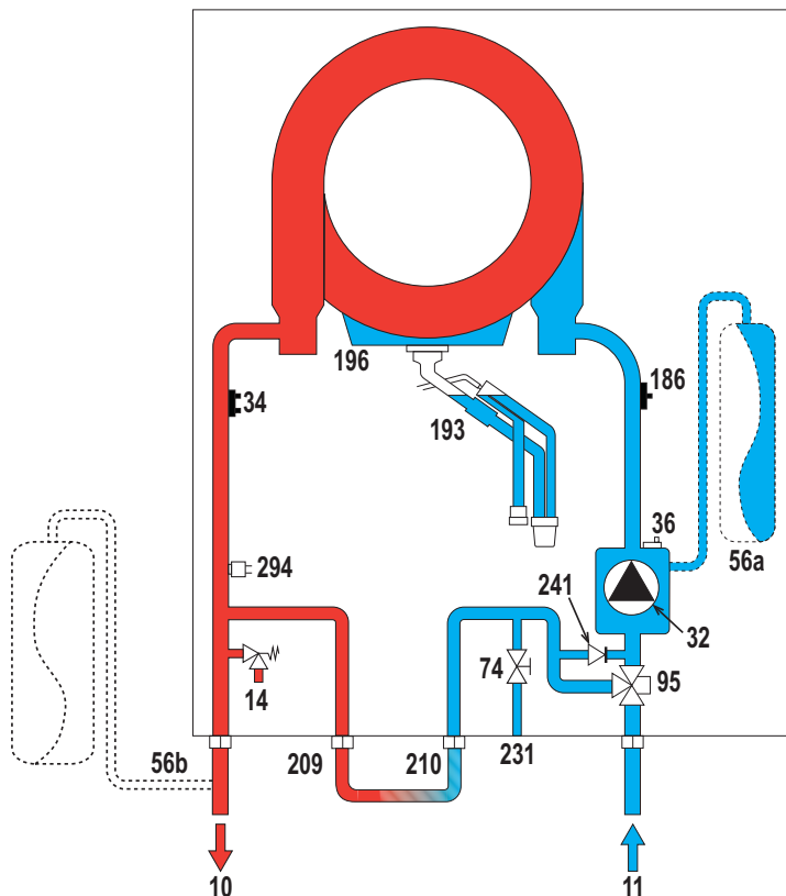
fig. 75- Circuitul hidraulic
