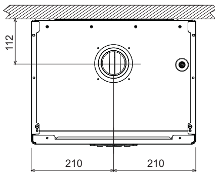
fig. 72- Vedere de sus
