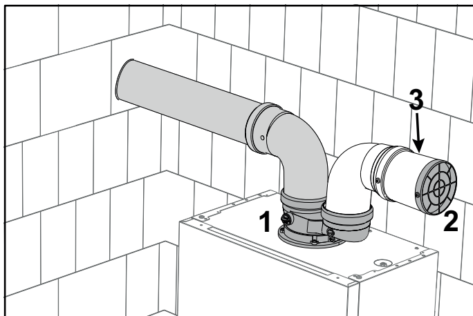
wygląd 48- Kratka ochronna
