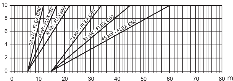
fig. 40- Gráfico para seleccionar el parámetro chimenea
