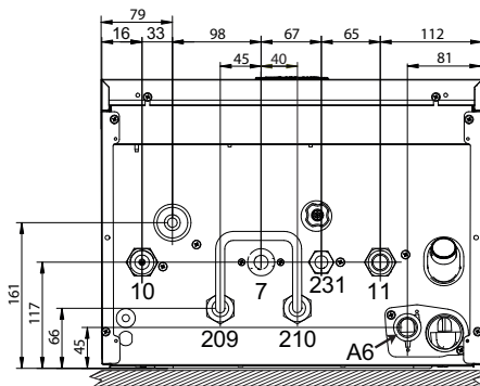
εικ. 73- Άνωψη
