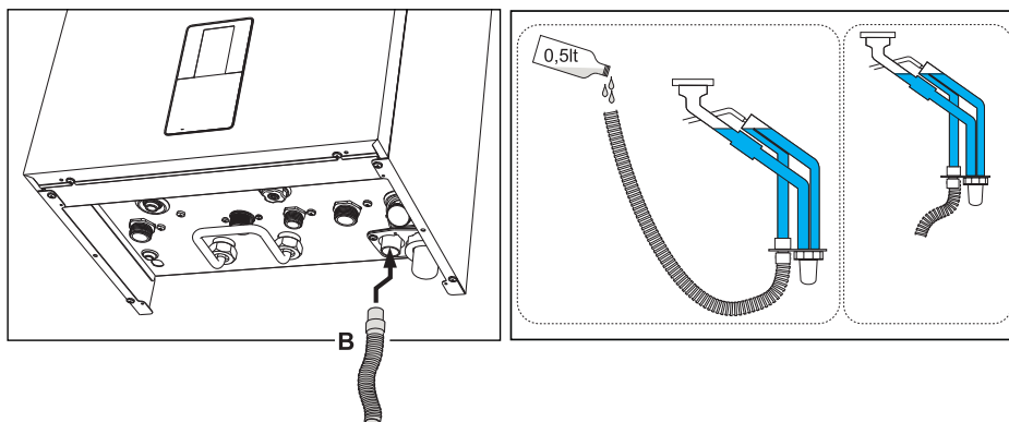
fig. 51- Conexión de la descarga de condensado
