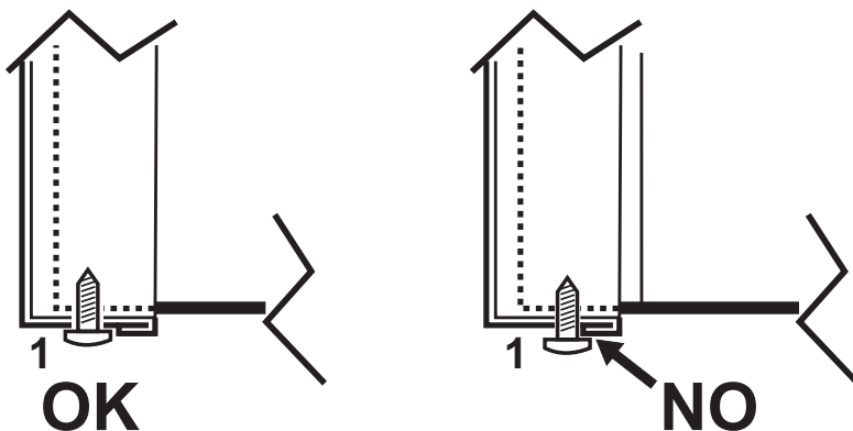
εικ. 56- Σωστή τοποθέτηση μπροστινού πίνακα
