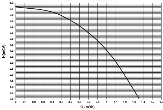
fig. 77- Carga hidrostática residual disponible en la instalación
