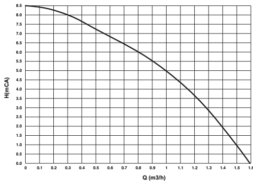
wygląd 78- Wysokość podnoszenia dostępna w instalacji
