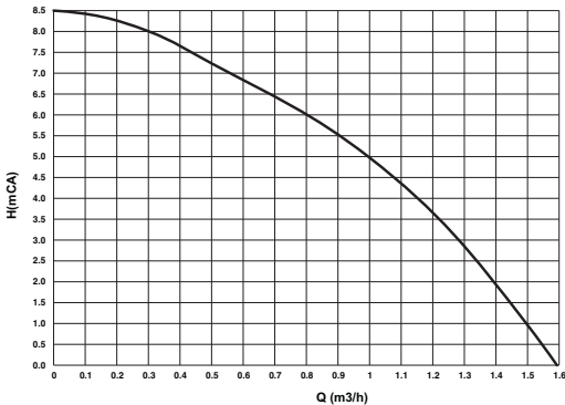
εικ. 78- Διαθέσιμο υπολειπόμενο μανομετρικό ύψος στην εγκατάσταση
