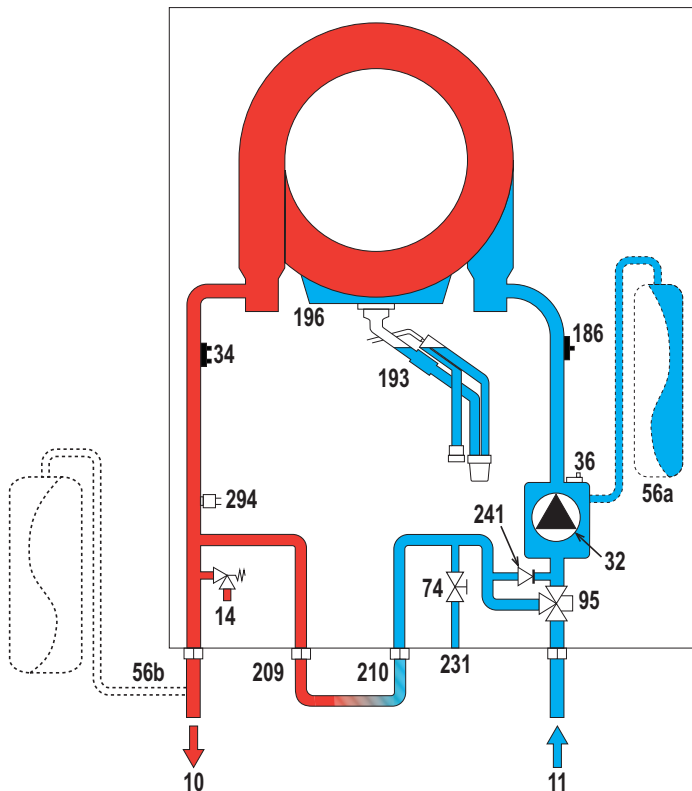
wygląd 75- Obieg wody
