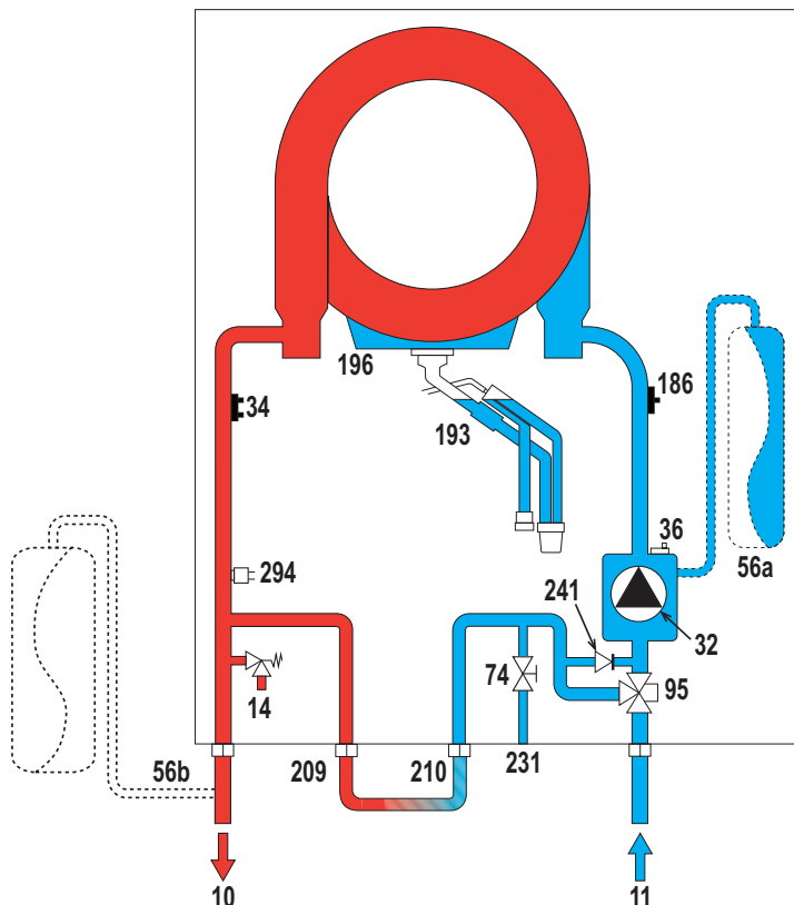
fig. 76 - Circuito idraulico
