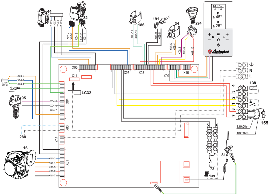
fig. 79- Wiring diagram
