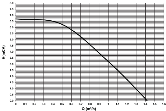
fig. 76- Înălțime de pompare reziduală disponibilă în instalație
