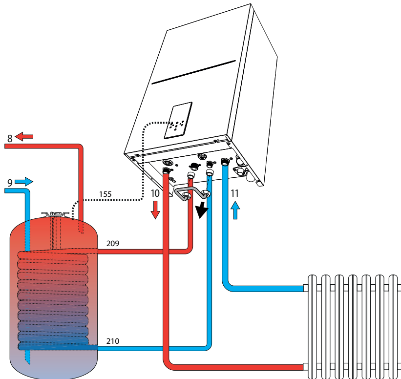
εικ. 28- Διάγραμμα σύνδεσης σε εξωτερικό μπόιλερ
