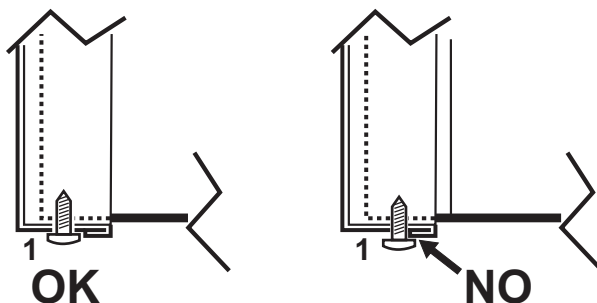
fig. 56- Poziția corectă a panoului frontal
