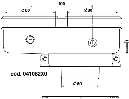
fig. 36 - Accessorio di partenza per condotti separati
