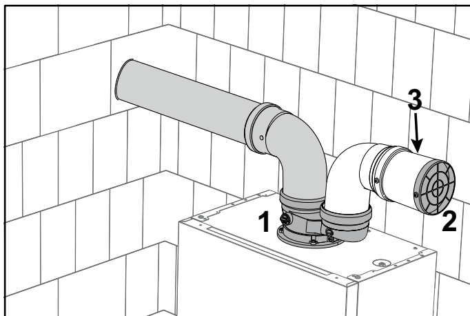
εικ. 48- Προστατευτική σχάρα
