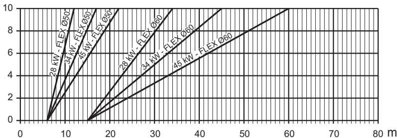
wygląd 40- Wykres wyboru parametrów przewodu spalinowego
