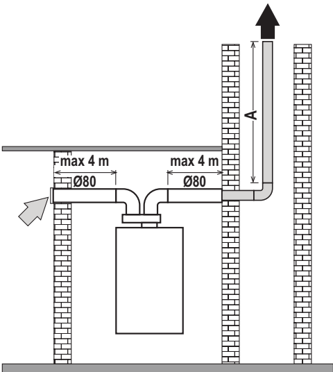
fig. 39 - Schema per solo intubamento con tubo flessibile
