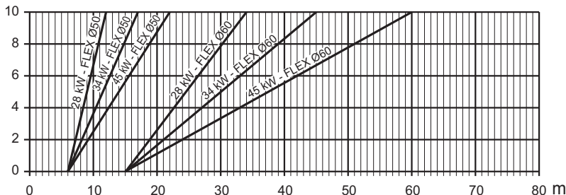
fig. 40 - Grafico per scelta parametro camino
