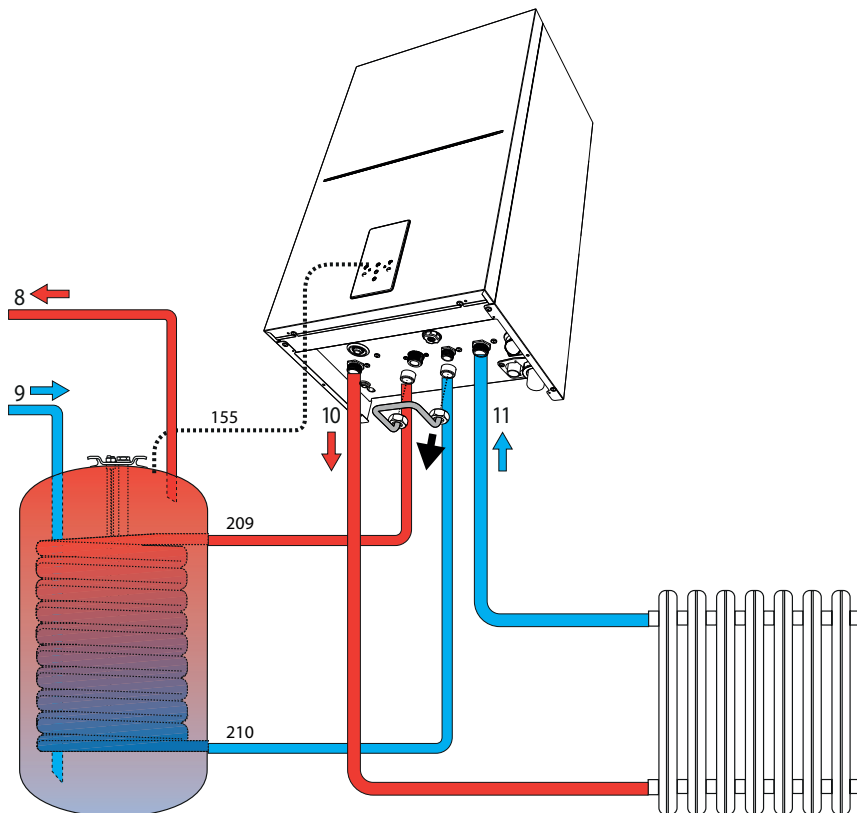
wygląd 28- Schemat podłączeń do zewnętrznego podgrzewacza
