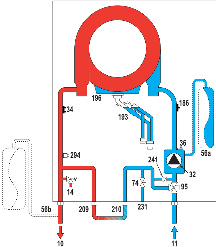
εικ. 75- Υδραυλικό κύκλωμα
