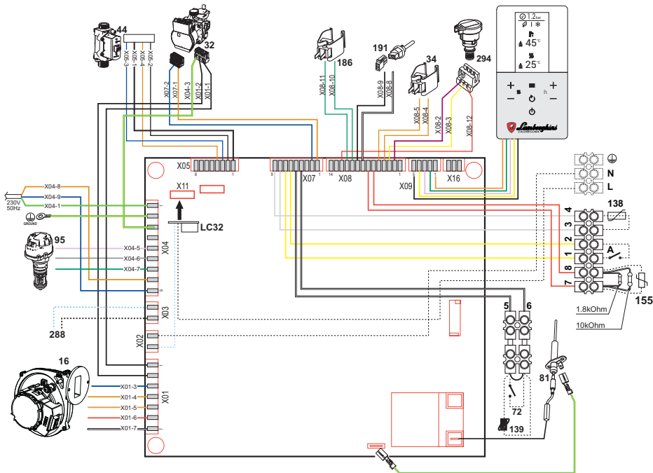
fig. 80 - Schema elettrico
