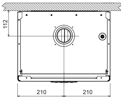
fig. 73 - Vista dall'alto
