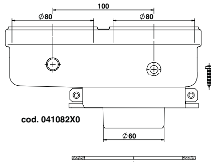
fig. 36- Accesorio inicial para conductos separados
