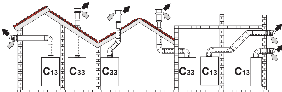
εικ. 31- Παραδείγματα σύνδεσης με ομοαξονικούς σωλήνες
