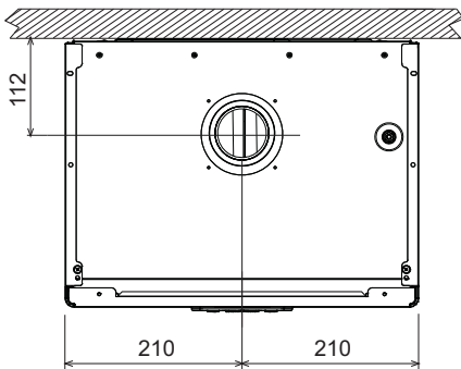
εικ. 72- Κάτωψη
