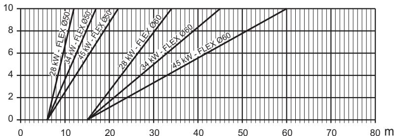
εικ. 40- Γραφικό για επιλογή παραμέτρου καπνοδόχου
