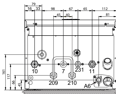
fig. 74 - Vista dal basso
