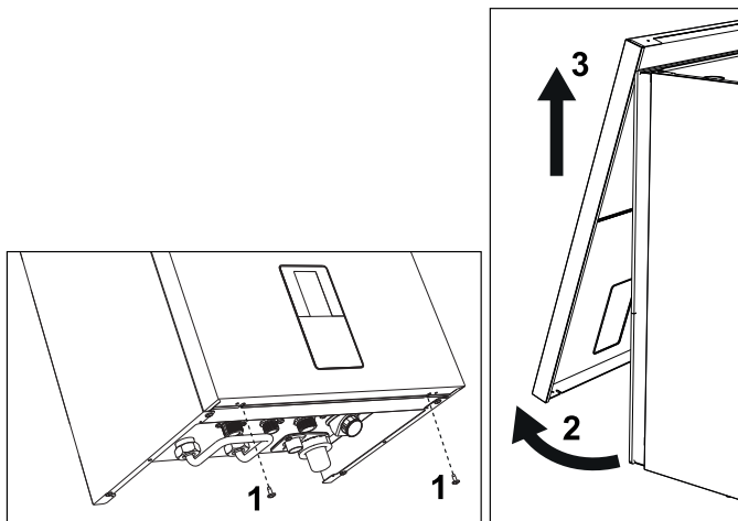
wygląd 55- Otwieranie panelu przedniego
