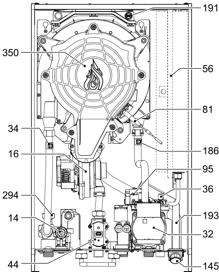
fig. 74- Vista general
