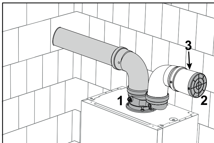
fig. 48- Protection grille
