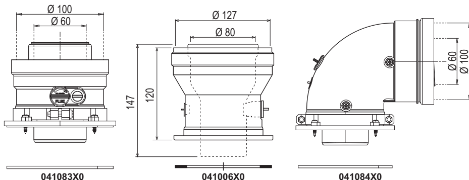
fig. 32 - Accessori di partenza per condotti coassiali
