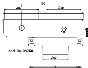
wygląd 36- Człon początkowy do montażu oddzielnych przewodów
