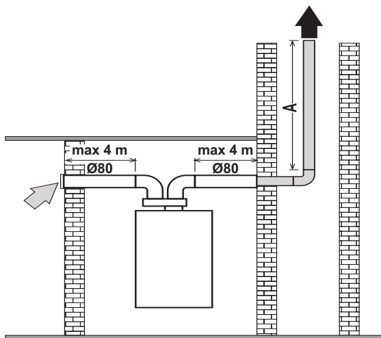
wygląd 39- Schemat dotyczy jedynie rozwiązania z elastycznym przewodem rurowym
