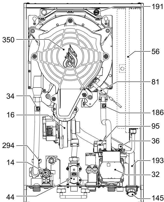
fig. 75 - Vista generale
