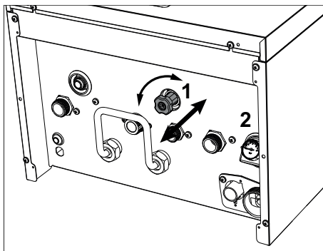
wygląd 26- Pokrętło napełniania
