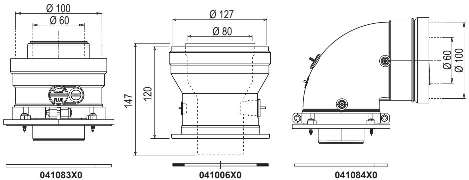
fig. 32- Accesorios iniciales para conductos coaxiales
