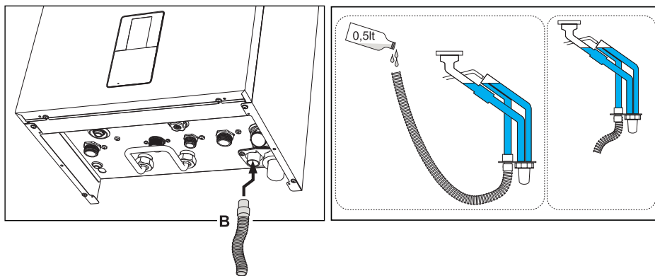
fig. 51 - Collegamento scarico condensa
