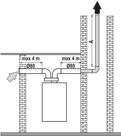
fig. 39- Schemă numai pentru tuburi flexibile
