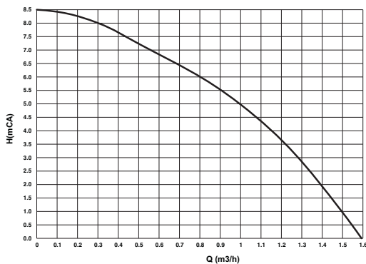
fig. 79 - Prevalenza residua disponibile all'impianto
