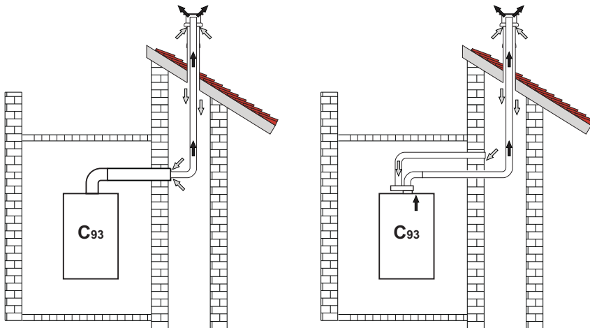
εικ. 43 Παραδείγματα σύνδεσης σε καπνοδόχους (⇨ = Αέρας / ⇨ = Καυσαέρια)
