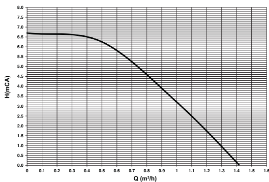
fig. 77 - Prevalenza residua disponibile all'impianto
