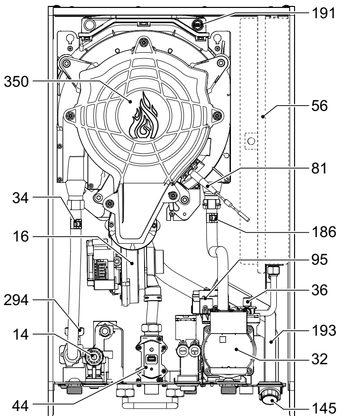
fig. 74- Vedere generală
