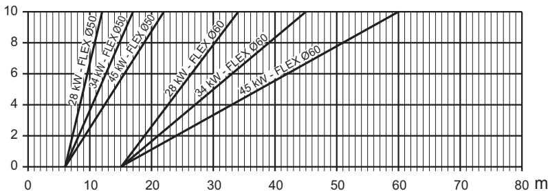
fig. 40- Chart for flue parameter choice
