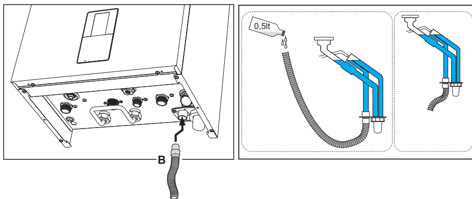
wygląd 51- Podłączenie spustu kondensatu
