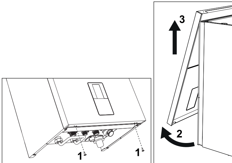
εικ. 55- Ανοιγμα μπροστινού πινάκα
