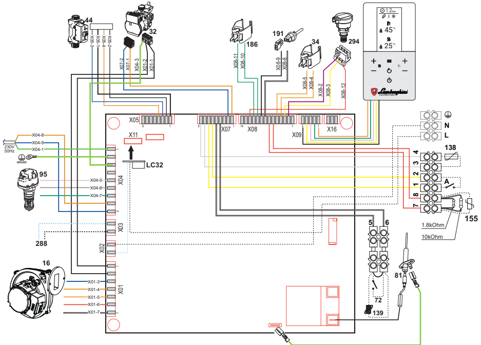
εικ. 79- Ηλεκτρολογικό διάγραμμα
