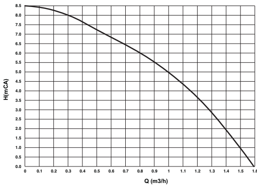
fig. 78- Carga hidrostática residual disponible en la instalación
