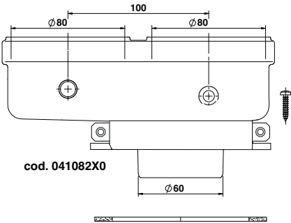
fig. 36- Accesoriu de pornire pentru conducte separate
