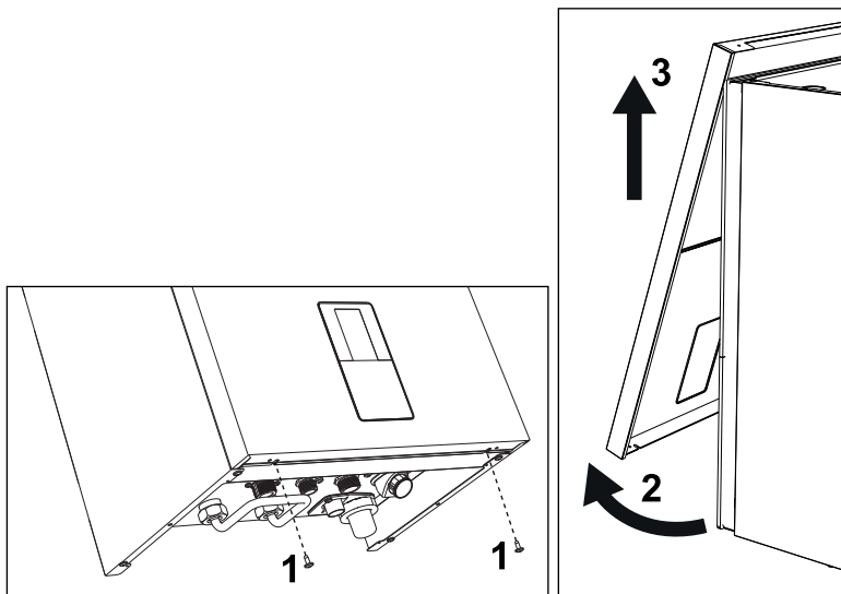
fig. 55- Apertura del panel frontal
