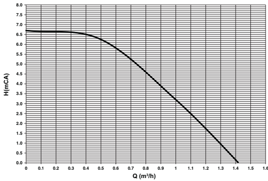
fig. 76- Carga hidrostática residual disponible en la instalación
