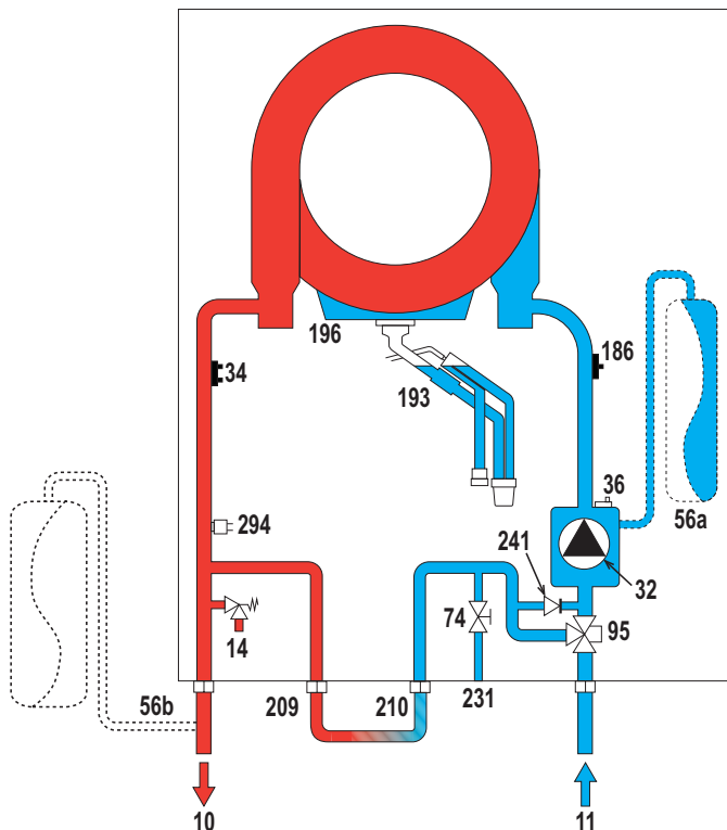
fig. 75- Circuito hidráulico
