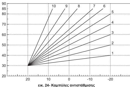
ΕΙΚ. 24- Καμπύλες αντιστάθμισης
