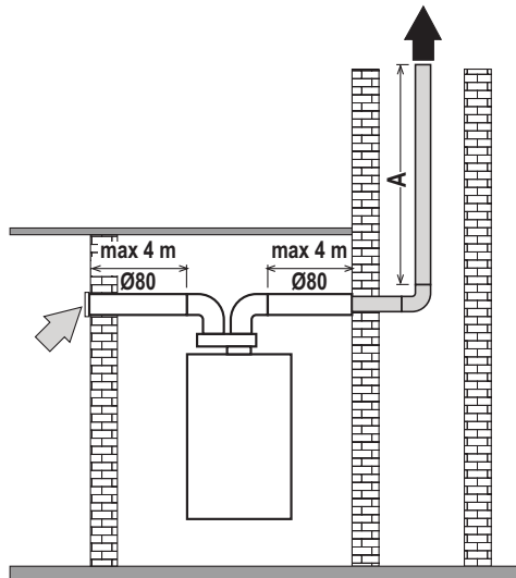
fig. 39- Esquema solo para entubamiento con flexible
