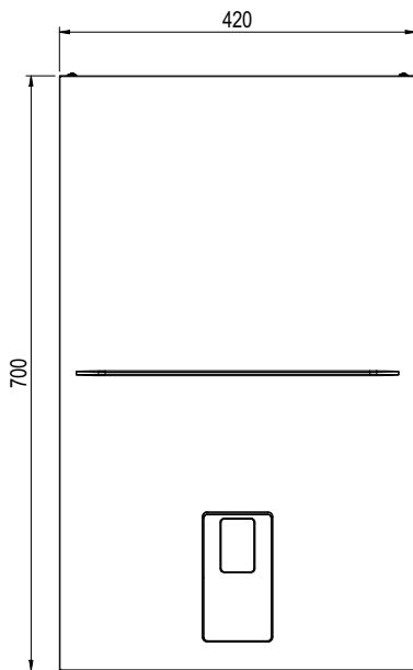
fig. 70- Vedere frontală
