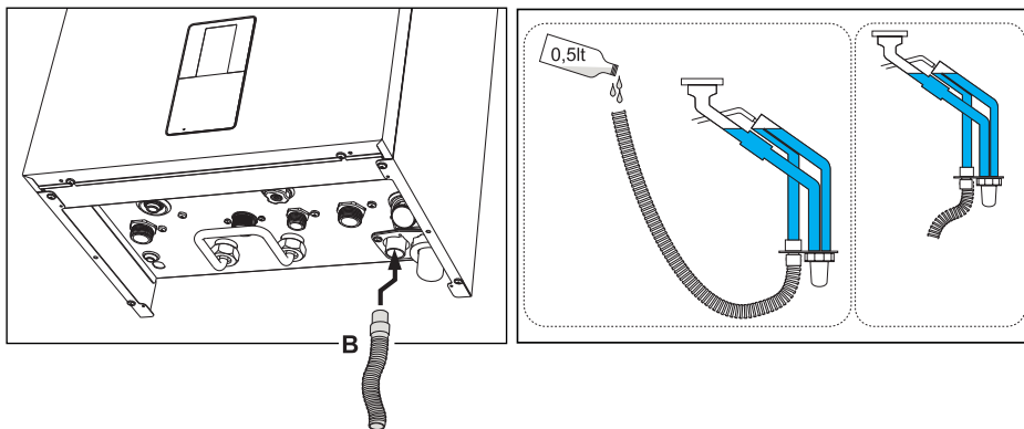
ΕΙΚ. 51- Σύνδεση εξαγωγής συμπυκνώματος
