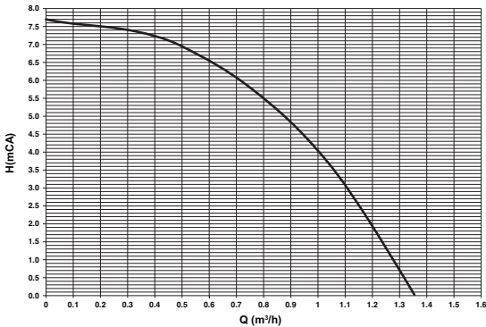
εικ. 77- Διαθέσιμο υπολειπόμενο μανομετρικό ύψος στην εγκατάσταση
