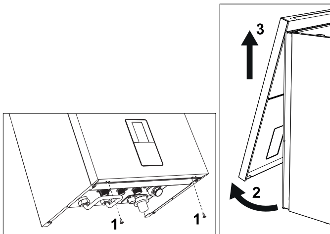
fig. 55- Deschiderea panoului frontal
