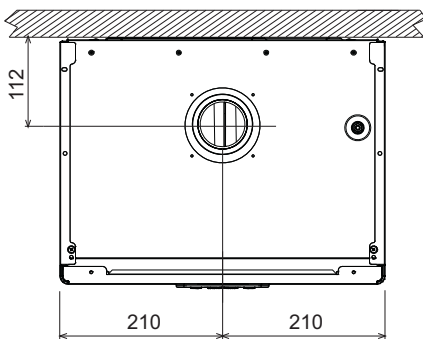
fig. 72- Vista superior
