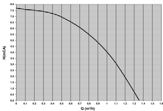
fig. 78 - Prevalenza residua disponibile all'impianto
