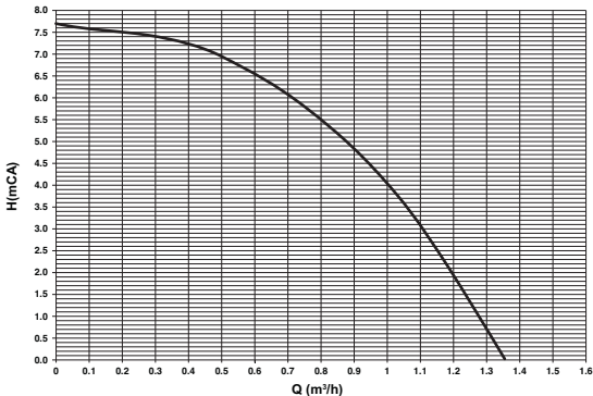
fig. 77- Înălțime de pompare reziduală disponibilă în instalație
