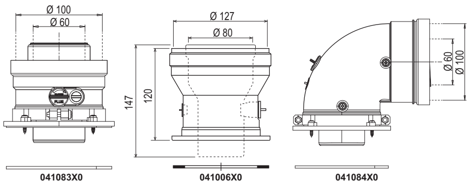
wygląd 32- Akcesoria wyjściowe do przewodów współosiowych
