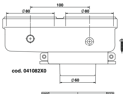
εικ. 36- Εξάρτημα σύνδεσης για ξεχωριστούς αγωγούς
